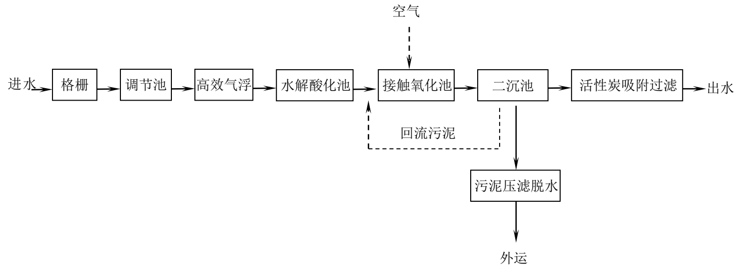
1、长春金赛药业股份有限公司天河街 72 号厂区污水处理设施工艺流程图
